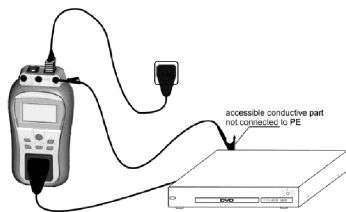
Test circuits for touch leakage current measurement Prüfschaltungen für die Berührungstrom-Messung
